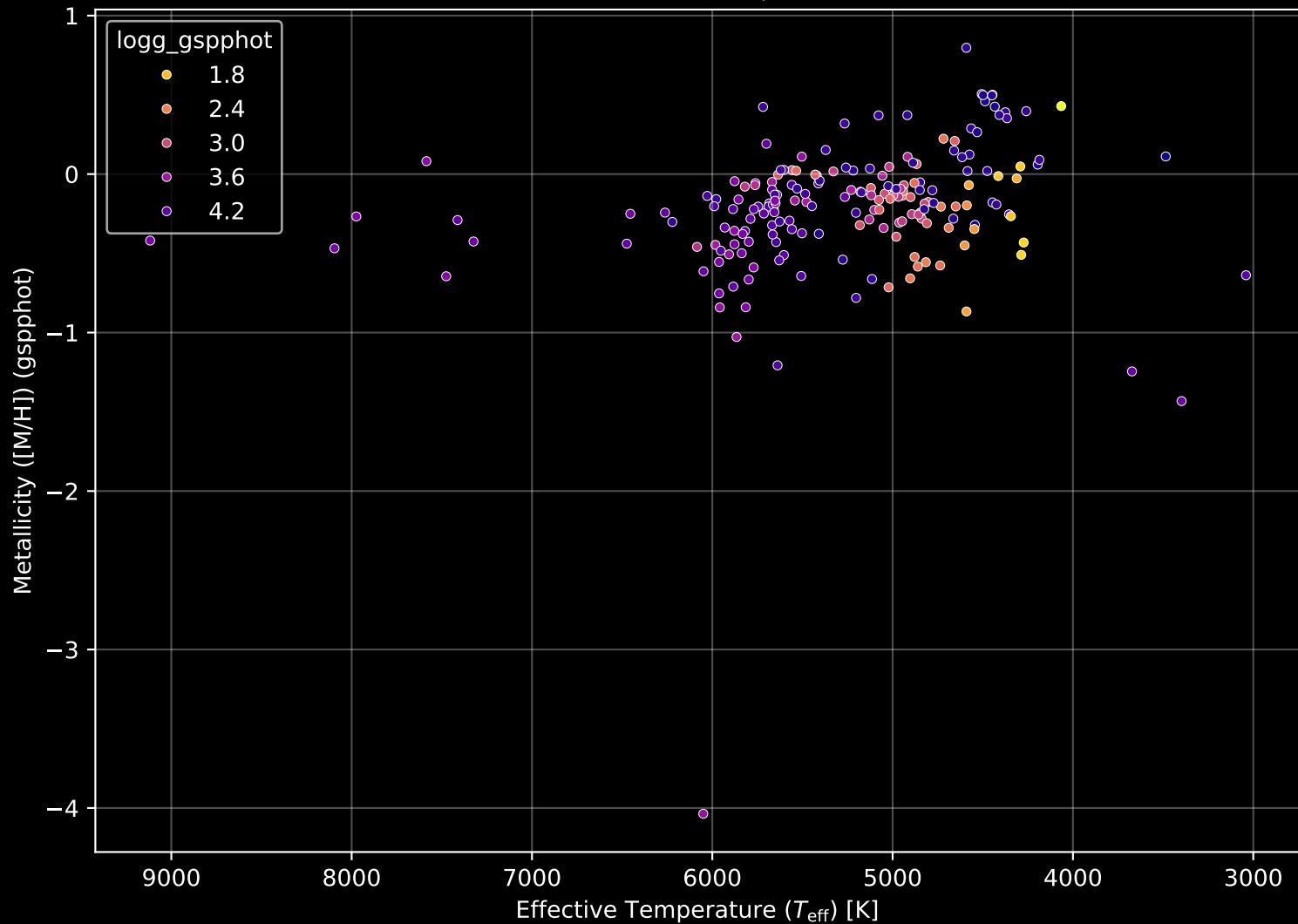
APOGEE DR17 Field: [177+32] Stellar Population Parameters (n= 197)
